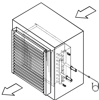
Антифризный термостат, установленный в возвратном коллекторе нагревателя.
