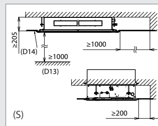
(размеры: мм)
