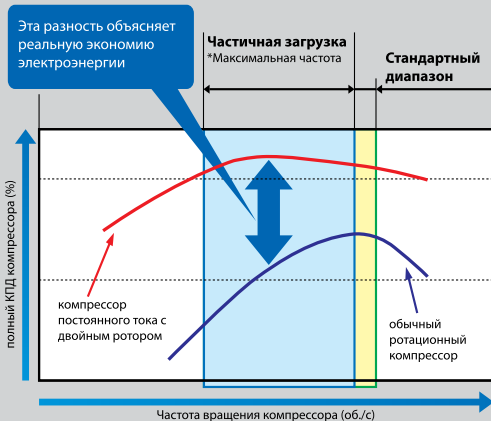
Сравнение компрессора постоянного тока с двойным ротором и обычного роторного компрессора
