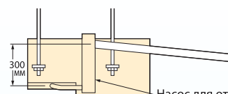
Насос для отвода конденсата
