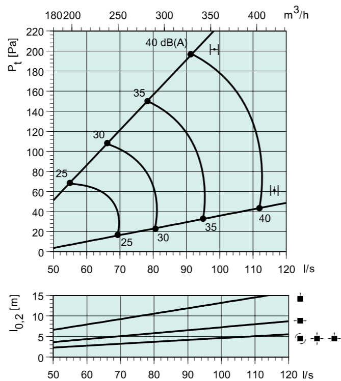
Sinus-A 250-L + PER 200
