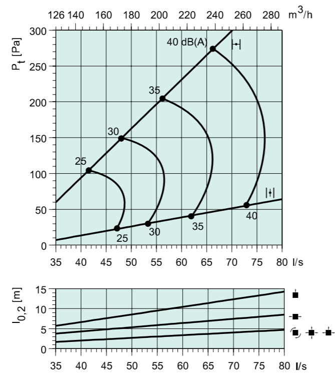
Sinus-A 200-L + PER 160
