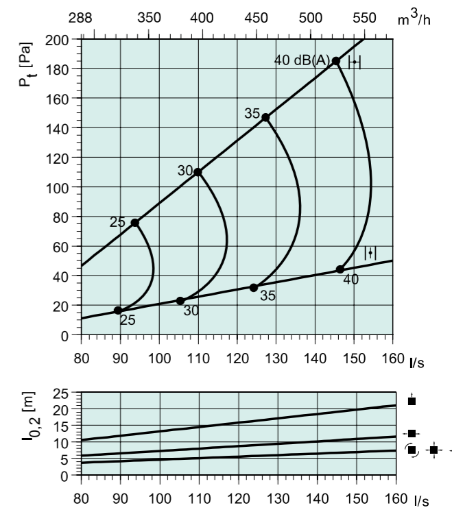
Sinus-A 315-L + PER 250
