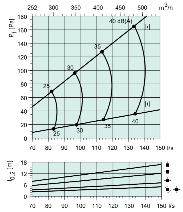
Sinus-A 315-S + PER 250
