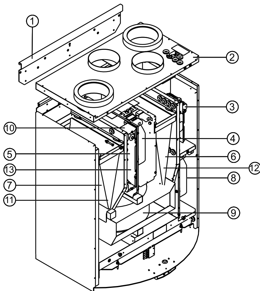
Рис. 13 Внутренние компоненты
