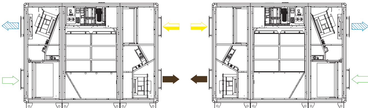
Левосторонний агрегат
