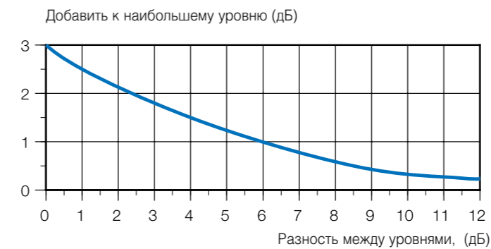
Рис. 5. Логарифмическое сложение
