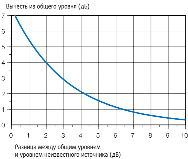
Рис. 6. Логарифмическое вычитание
