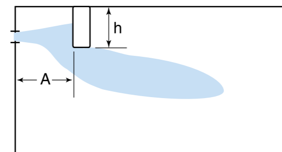
Рис. 17. Минимальное расстояние до препятствия
