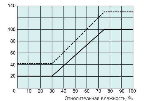
Расход воздуха, м³/ч при 100Па
