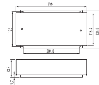
СОГЛАСОВАТЕЛЬ РАБОТЫ SERI-PARA I/O ДЛЯ КАЖДОГО ВНУТРЕННЕГО БЛОКА (CZ-CAPBC2)
