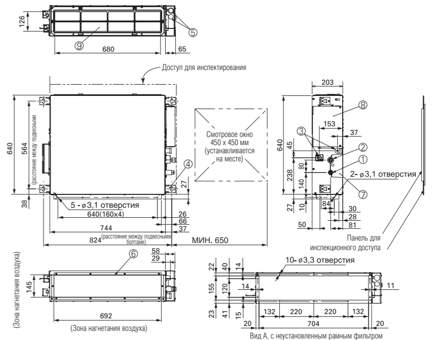
Вид А, с неустановленным рамным фильтром Размеры: мм
