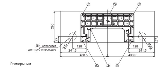
Размеры: мм
