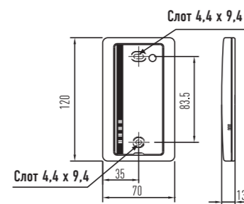
ОТДЕЛЬНЫЙ ПРИЕМНИК СИГНАЛОВ БЕСПРОВОДНОГО ПУЛЬТА ДУ (CZ-RWSC2)
