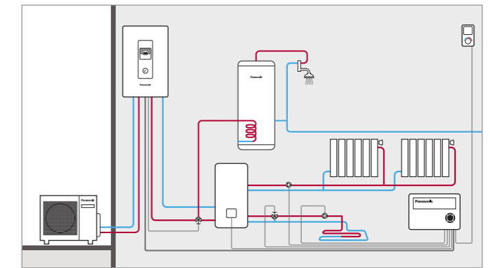
Управление температурой в 2 зонах + ECS с PAW-HPM12ZONE-U
