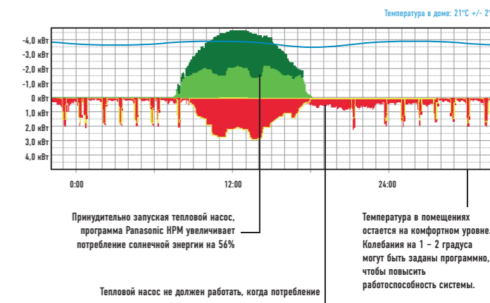
Типичный график потребления и производства электроэнергии С ИСПОЛЬЗОВАНИЕМ Panasonic HPM
