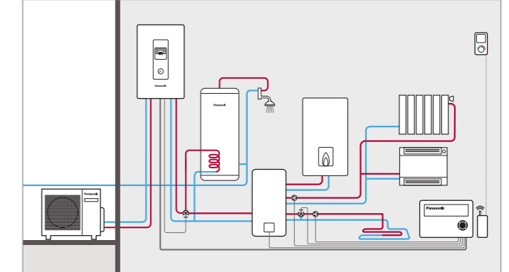
Управление тепловым насосом + бойлер и система DHW с PAW-HPM12ZONELCD-U
