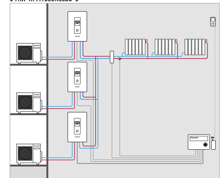
3 тепловых насоса, управляемых в каскадном режиме, с PAW-HPM12ZONELCD-U
