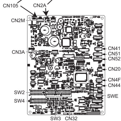
Плата управления внутреннего блока
