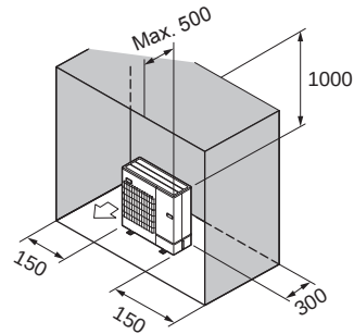
Fig. 2-12
