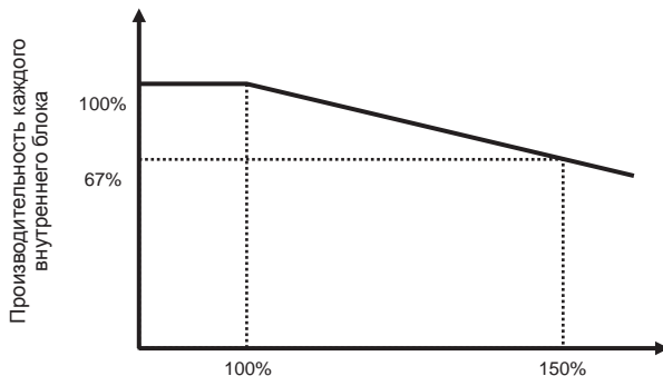
Соотношение общей производительности внутренних блоков и производительности наружного блока.
