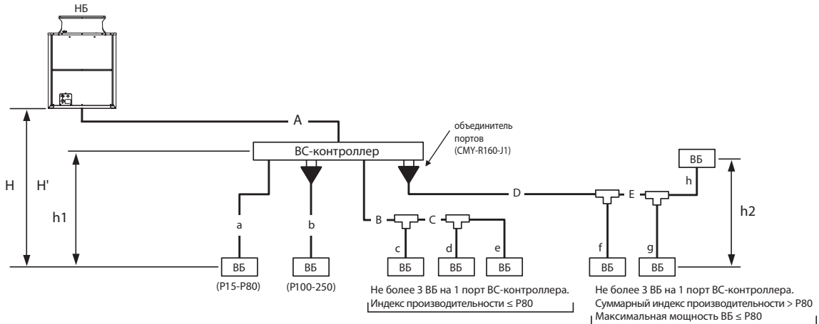
Рис. 7-1A. Схема фреопроводов
