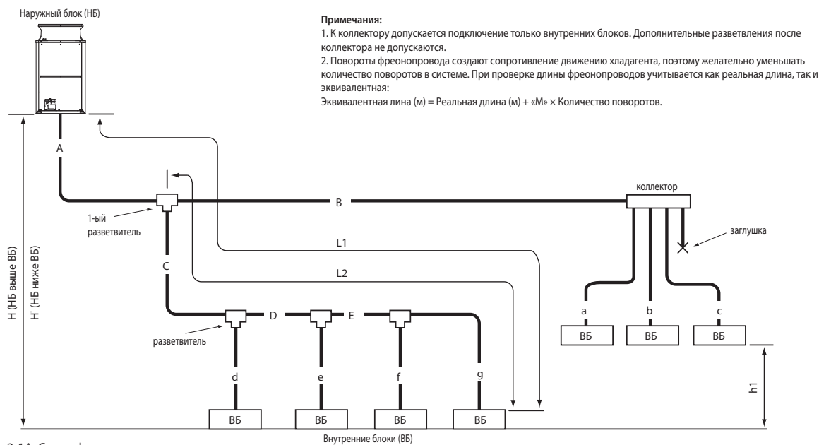
Рис. 2-1А. Схема фреоноводов
