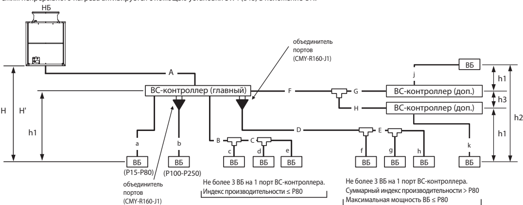
Рис. 7-1Б. Схема фреопроводов
