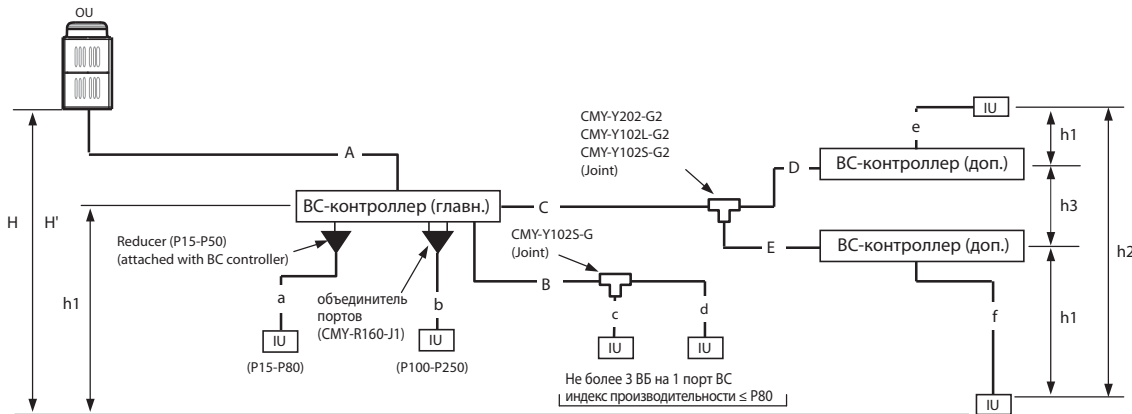
Рис. 8-2-2. Схема фреопроводов
