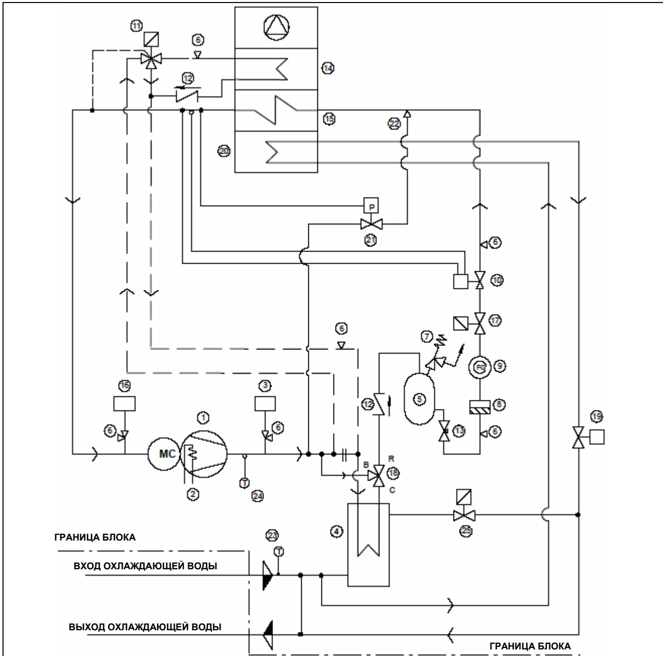
Рис. 8. Liebert Hiross HPM Sxx U/O F
