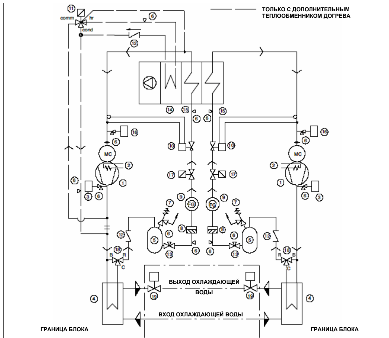
Рис. 6. Liebert Hiross HPM M34 - 66 U/O W
