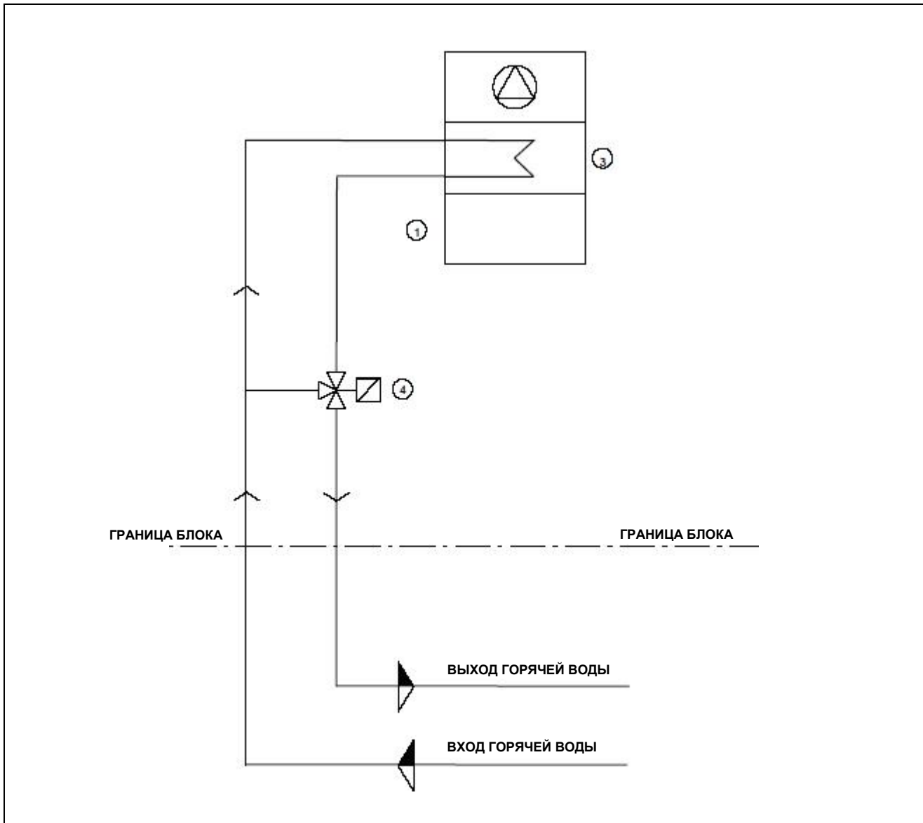
Рис. 1. Теплообменник догрева горячей водой - опция
