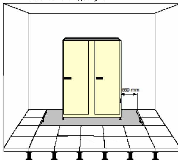
Рис. j – Снятие плиток фальшпола для безопасного доступа
