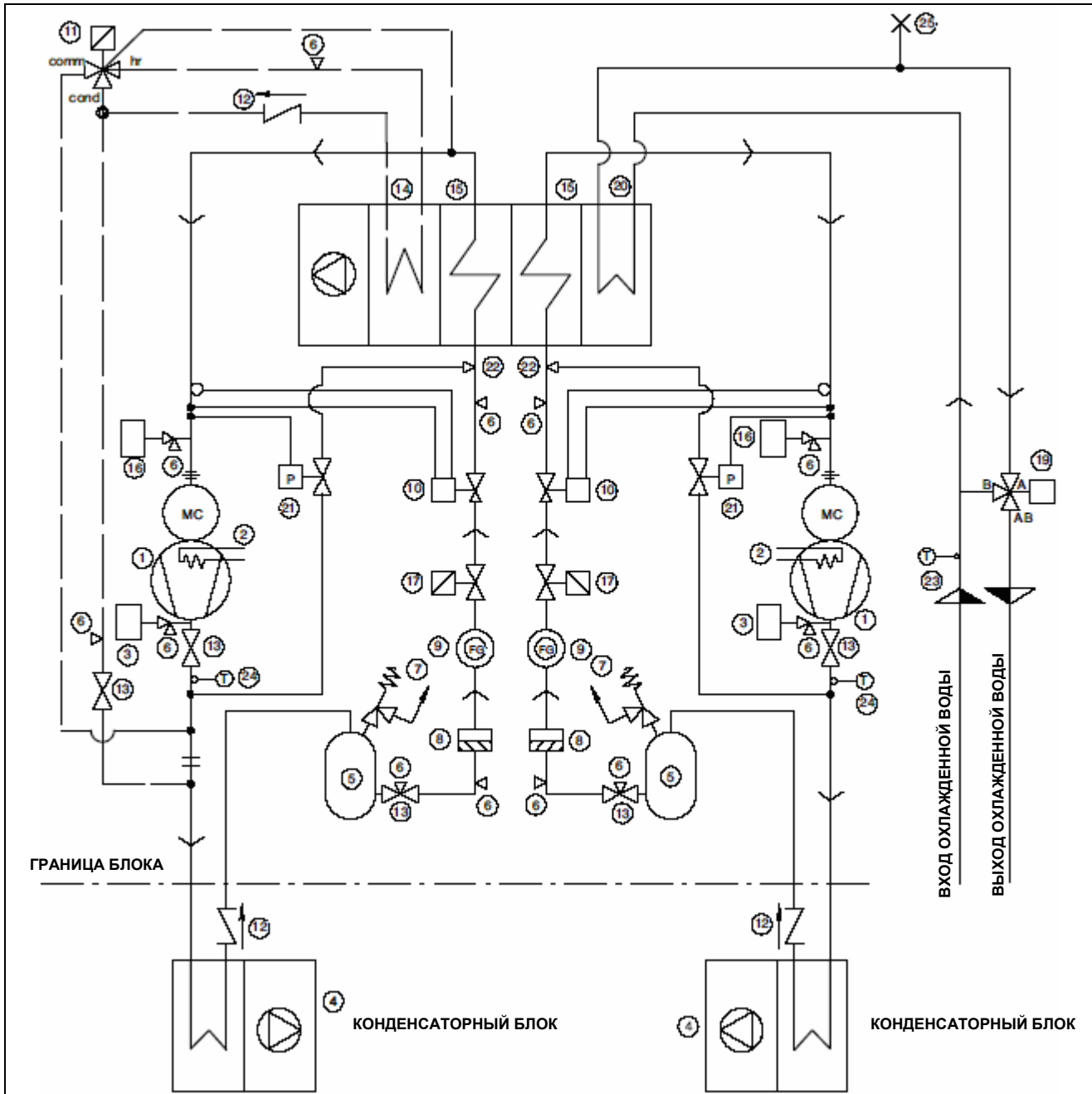
Рис. 13. Liebert Hiross HPM M34 - 58 U/O D
