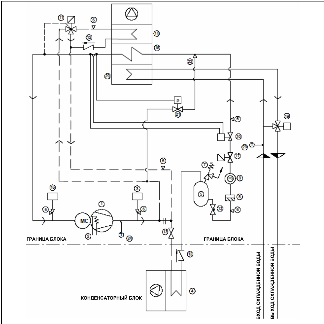
Рис. 12. Liebert Hiross HPM Sxx U/O D, M25 - 47 U/O D
