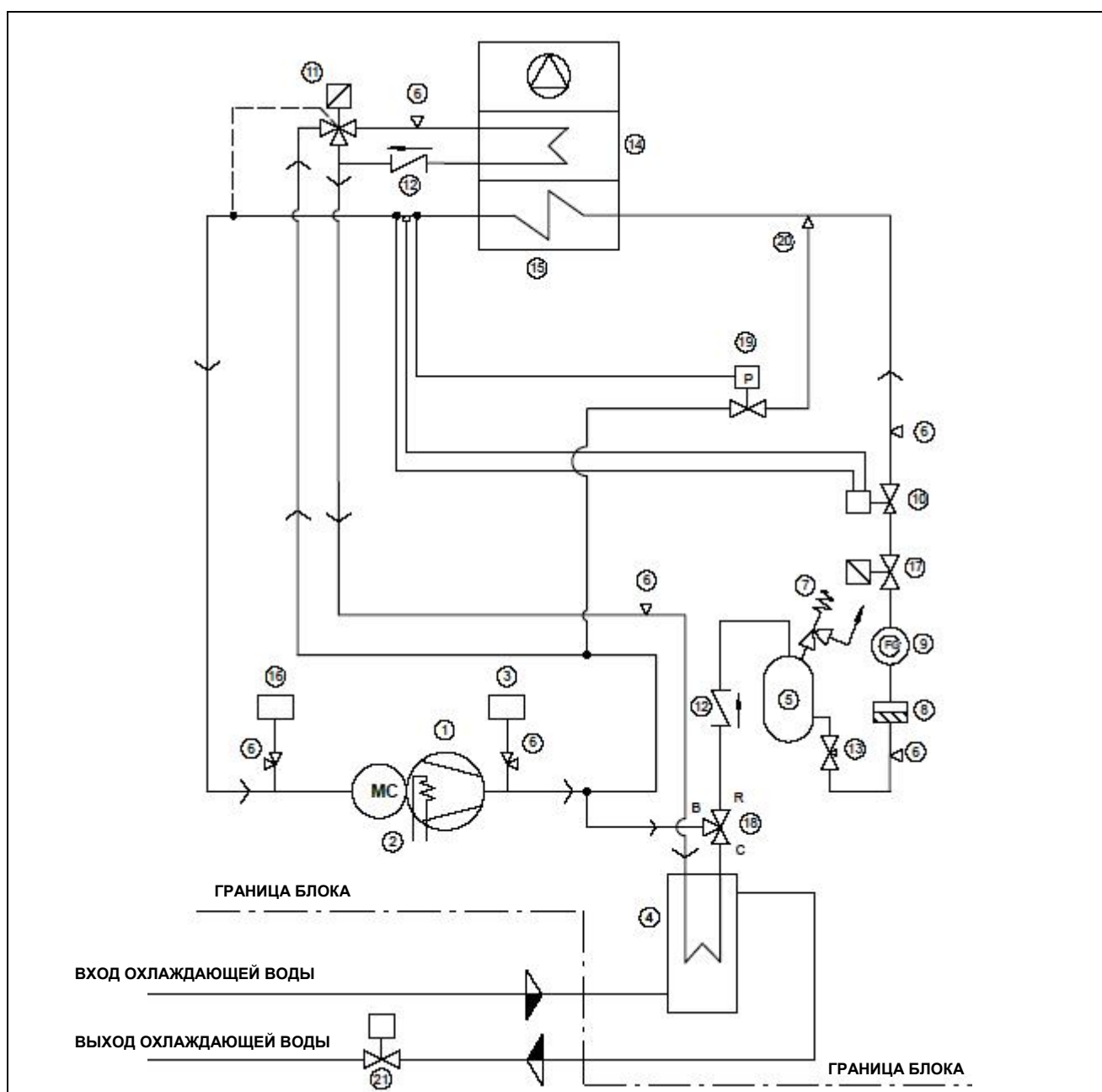
Рис. 20. Liebert Hiross HPM Sxx KW
