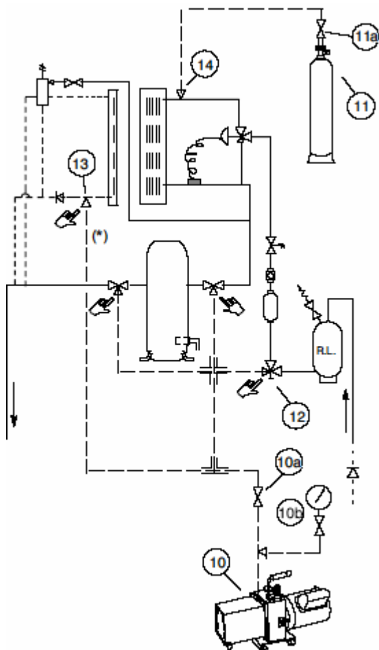
Рис. с – Подключение насоса и заправочного цилиндра для вакуумирования и заправки контура хладагентом
