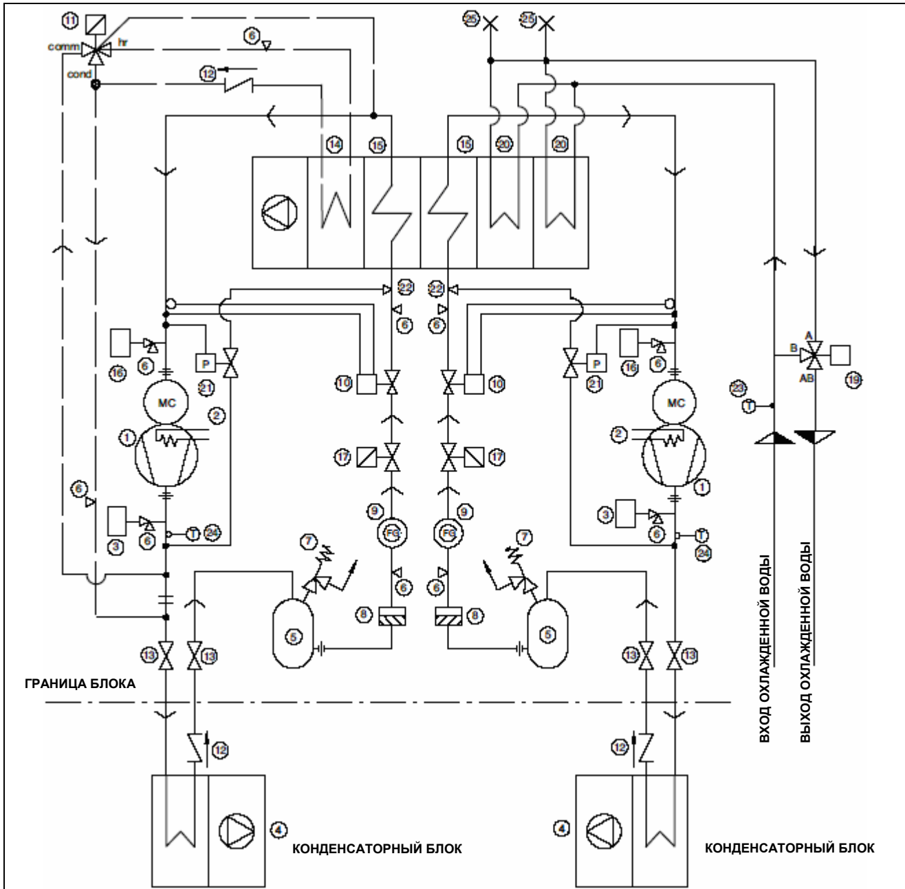
Рис. 14. Liebert Hiross HPM L83 U D
