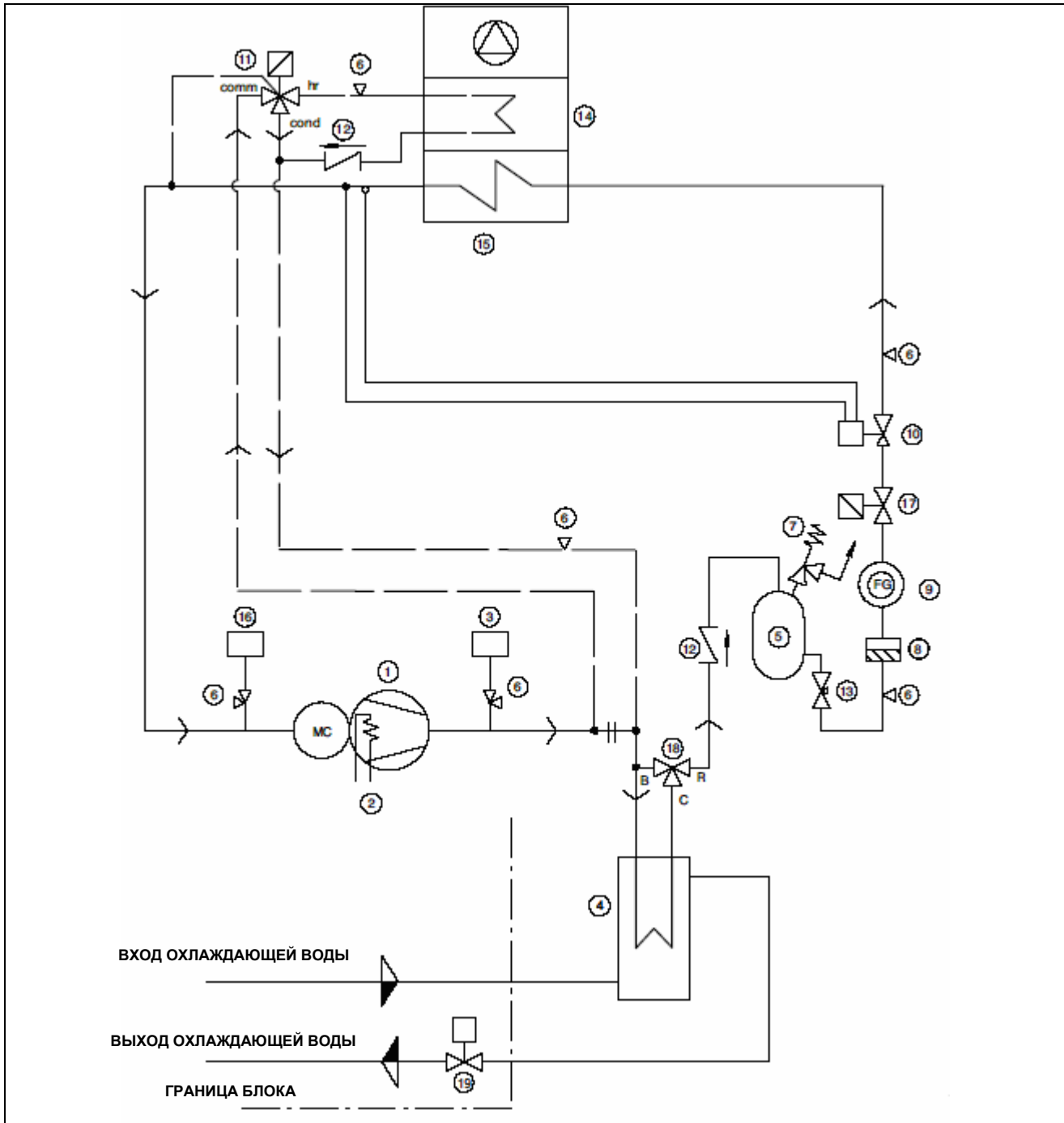
Рис. 5. Liebert Hiross HPM M25 - 47 U/O W
