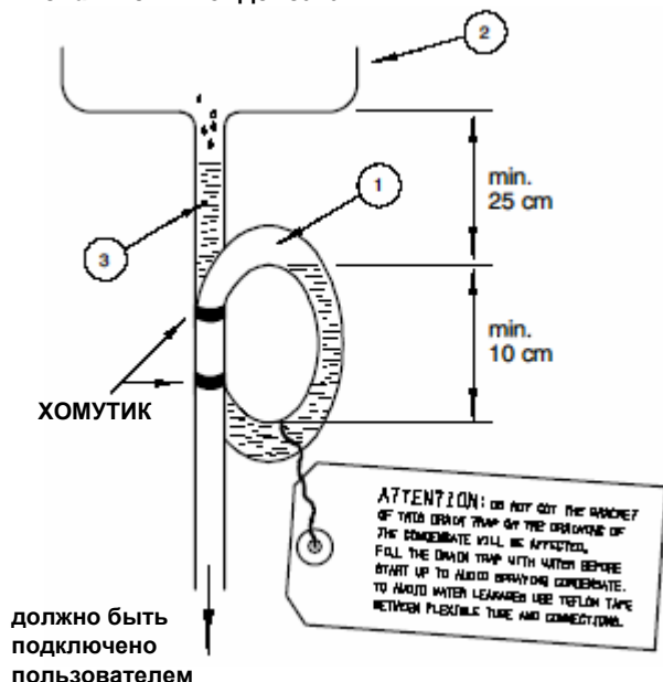
Рис. d – Слив конденсата
