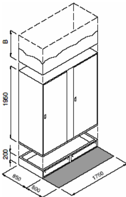
Рис. 3. Внешние размеры Зона обслуживания M31 - 66
