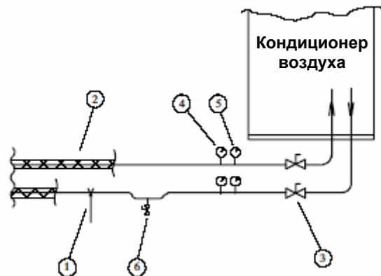
Рис. e – Контур охлажденной воды
