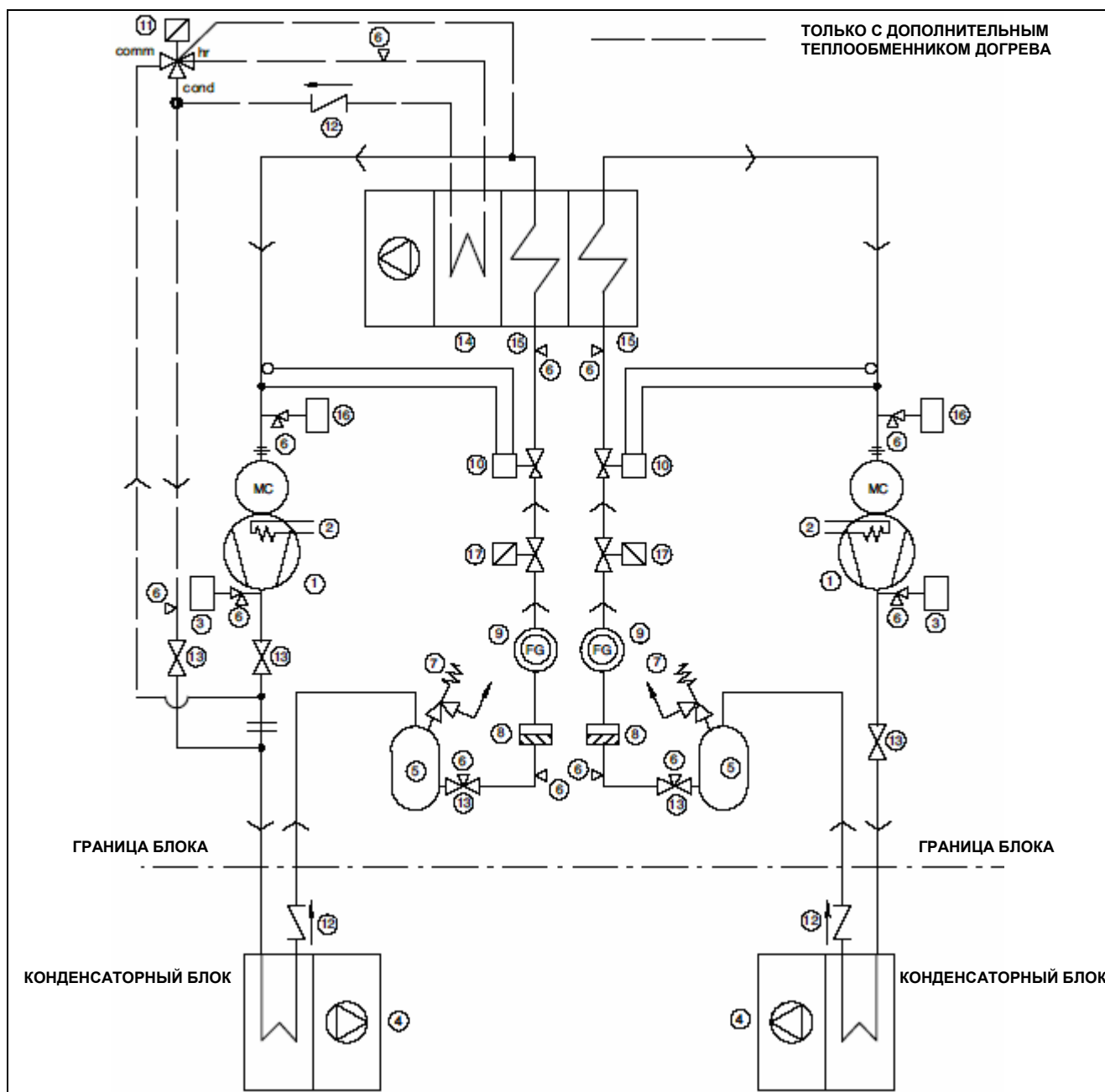
Рис. 2. Liebert Hiross HPM M34 – 66 U/O A
