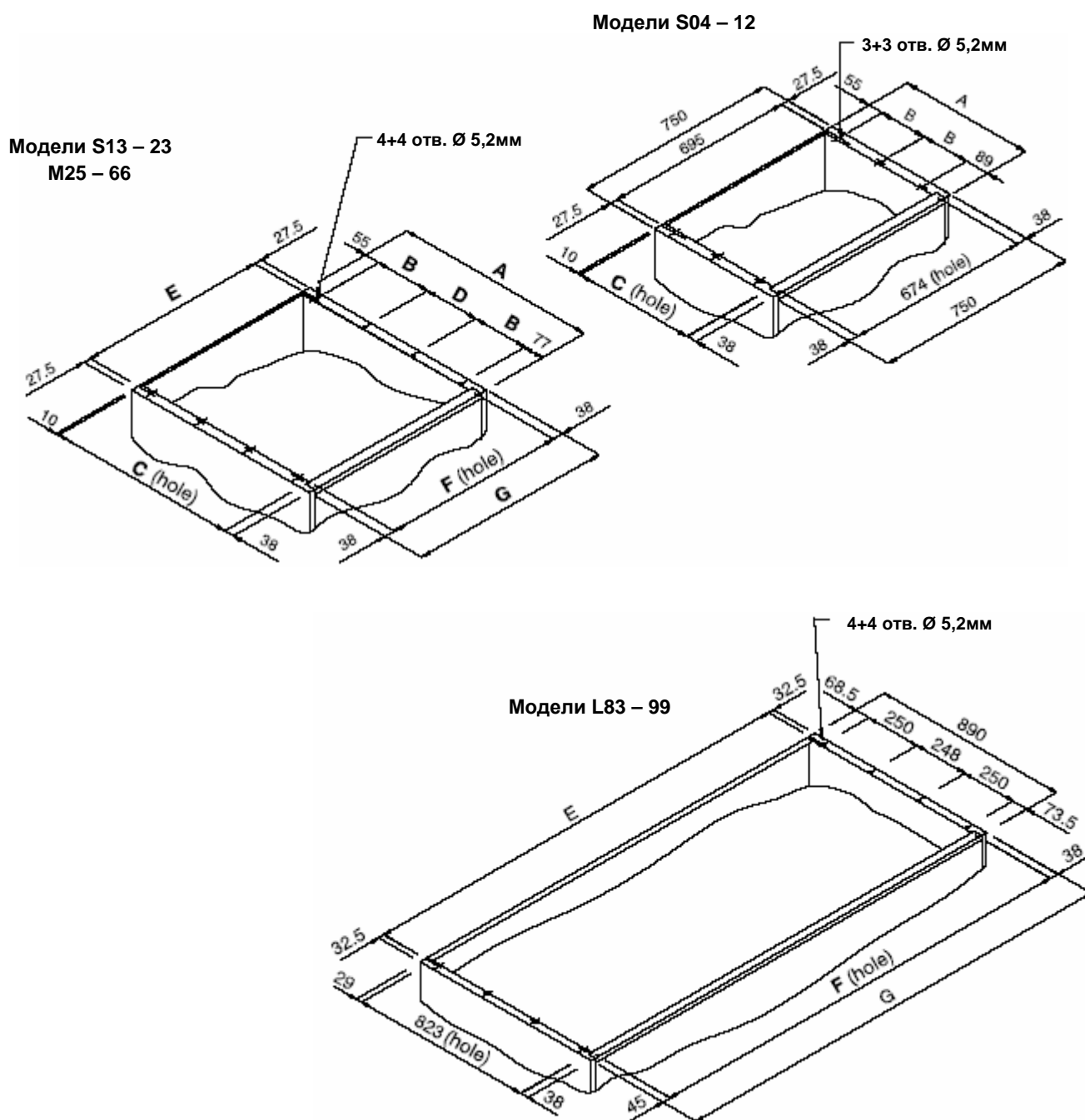
Рис. 5. Вход и выход воздуха – отверстия для подсоединения пленума
