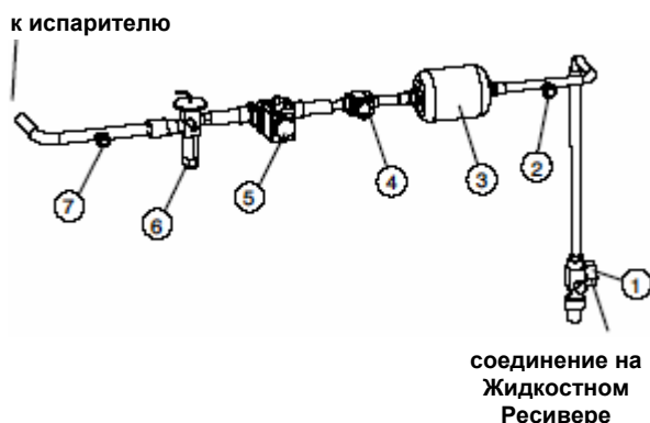
Рис. i – Элементы хладагентного трубопровода
