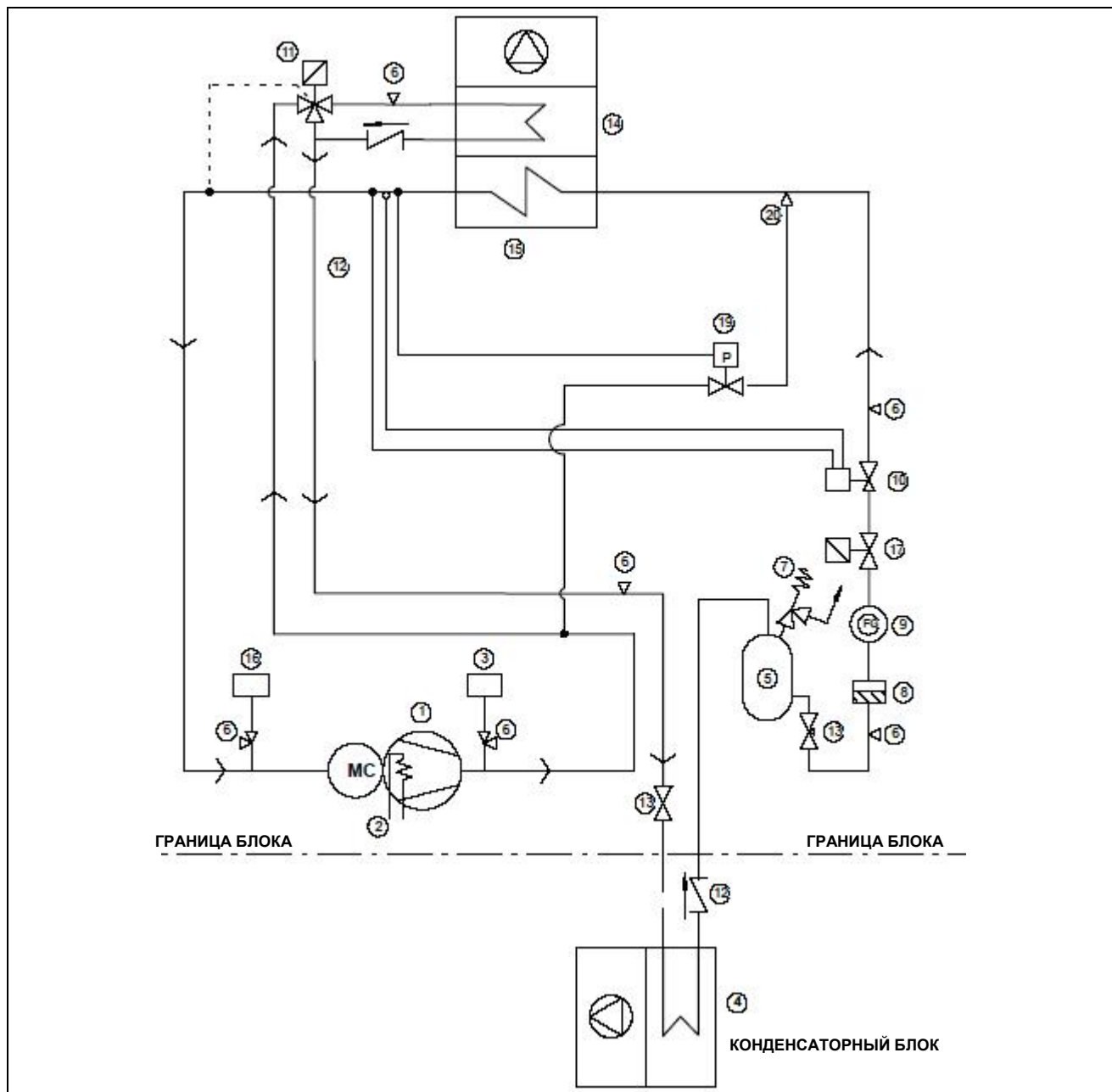
Рис. 19. Liebert Hiross HPM Sxx KA, M25 KA
