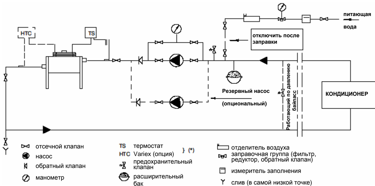
Рис. f – Рекомендуемая установка Драйкулера
