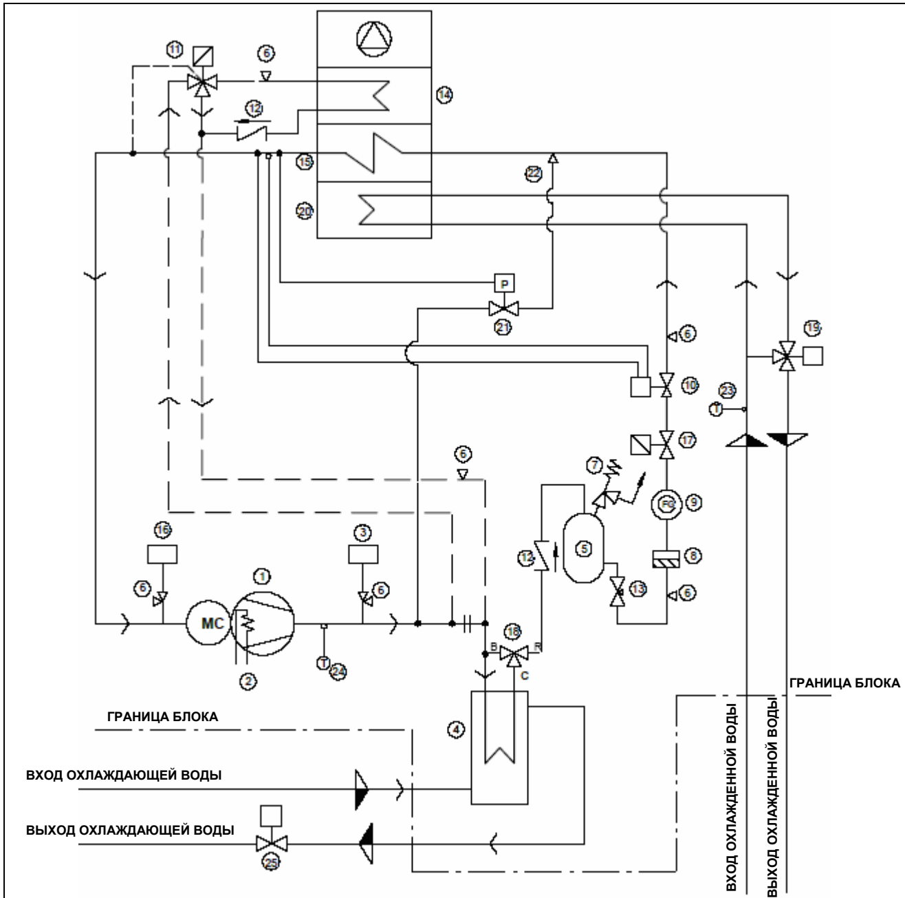
Рис. 16. Liebert Hiross HPM M25 - 47 U/O H
