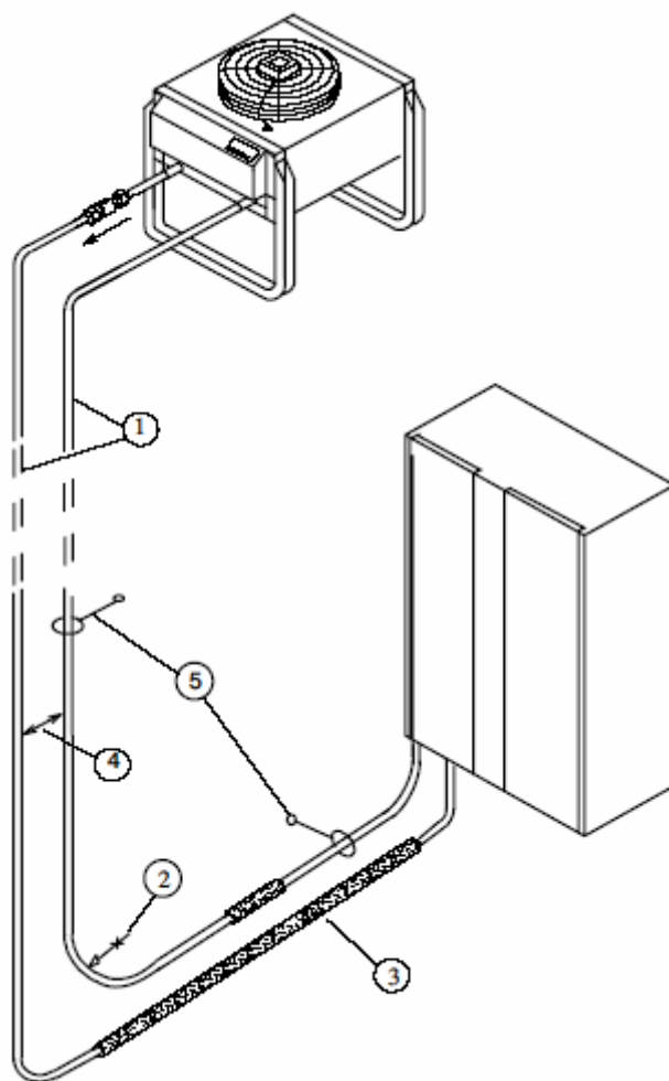
Рис. b – Рекомендуемая схема прокладки труб
