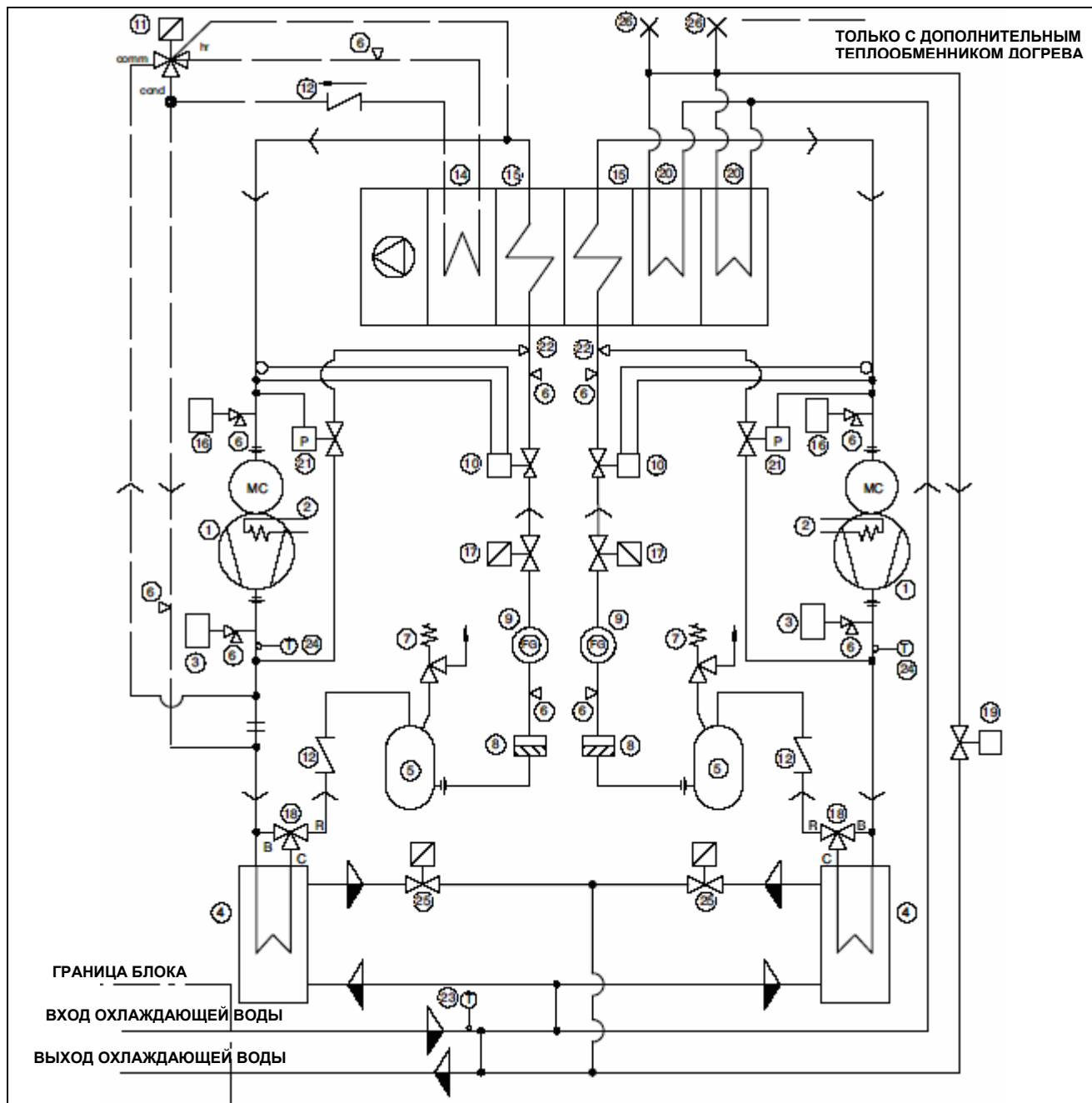
Рис. 11. Liebert Hiross HPM L83 U F
