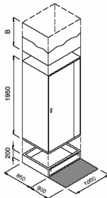
Рис. 4. Внешние размеры Зона обслуживания L83 – 99
