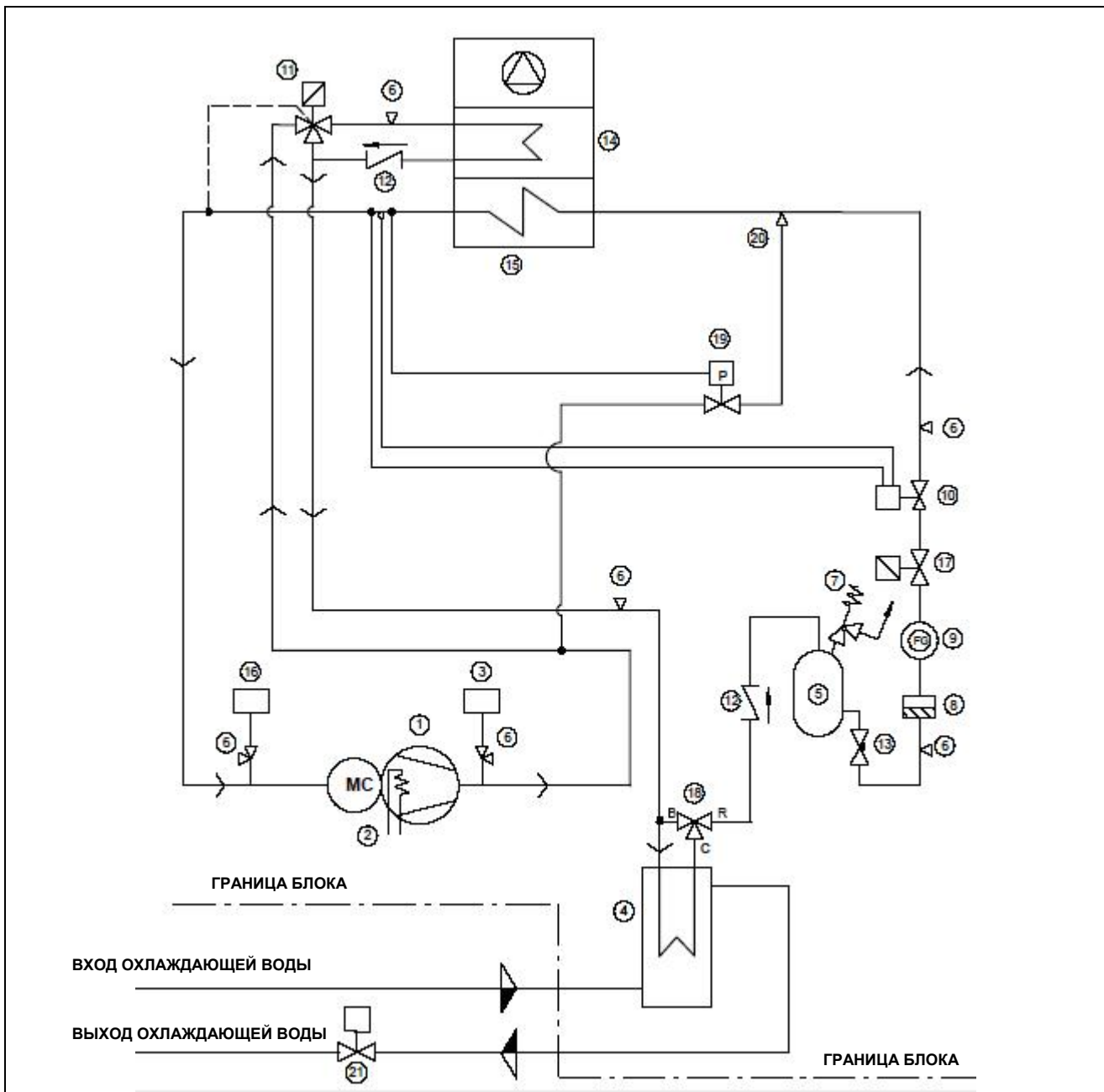
Рис. 21. Liebert Hiross HPM M25 KW
