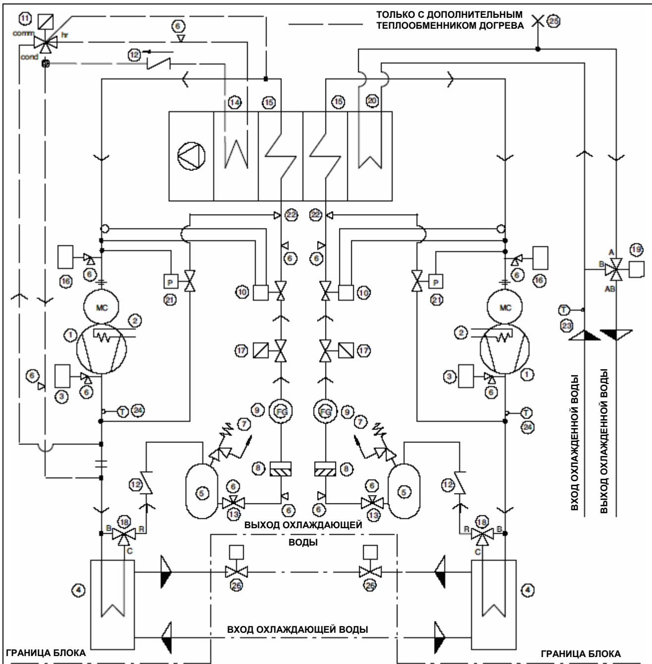
Рис. 17. Liebert Hiross HPM M34 - 58 U/O H
