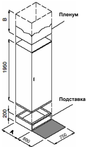
Рис. 3. Внешние размеры Зона обслуживания M31 - 66
