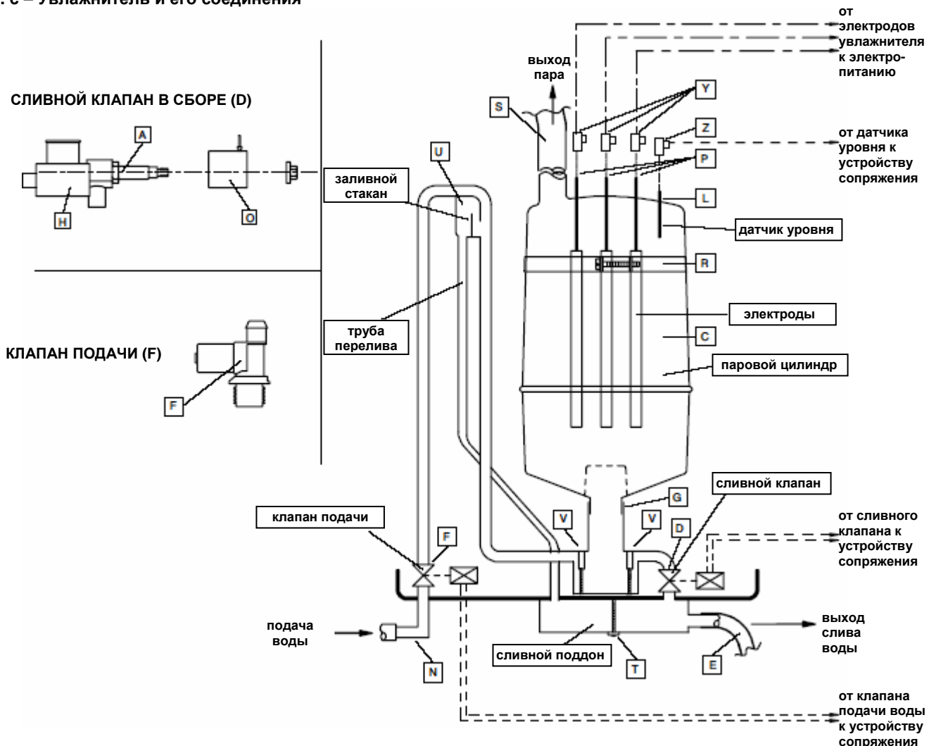
Рис. с – Увлажнитель и его соединения
