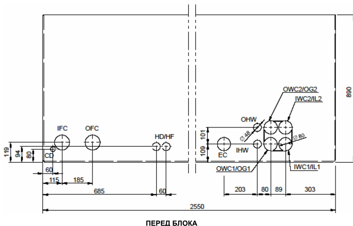
Рис. 6. Хладагентные, водяные и электрические соединения Liebert Hiross HPM L83 – 99
