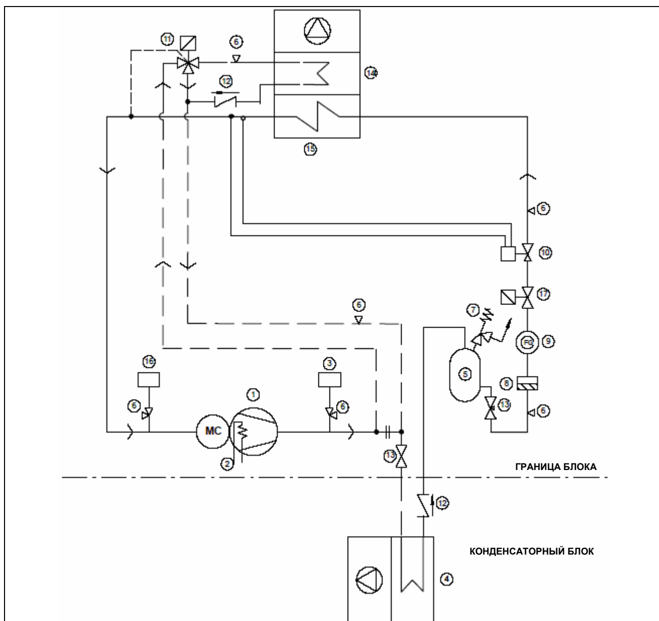
Рис. 1. Liebert Hiross HPM Sxx U/O A, M25 – 47 U/O A
