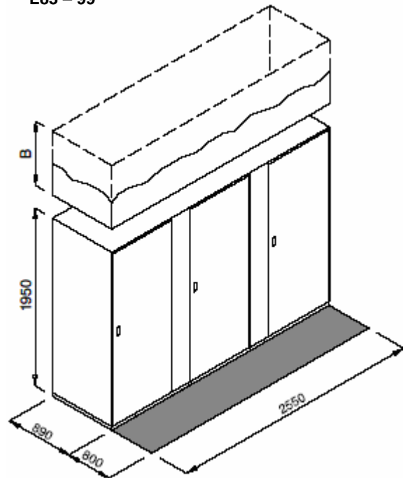
Рис. 4. Внешние размеры Зона обслуживания L83 – 99
