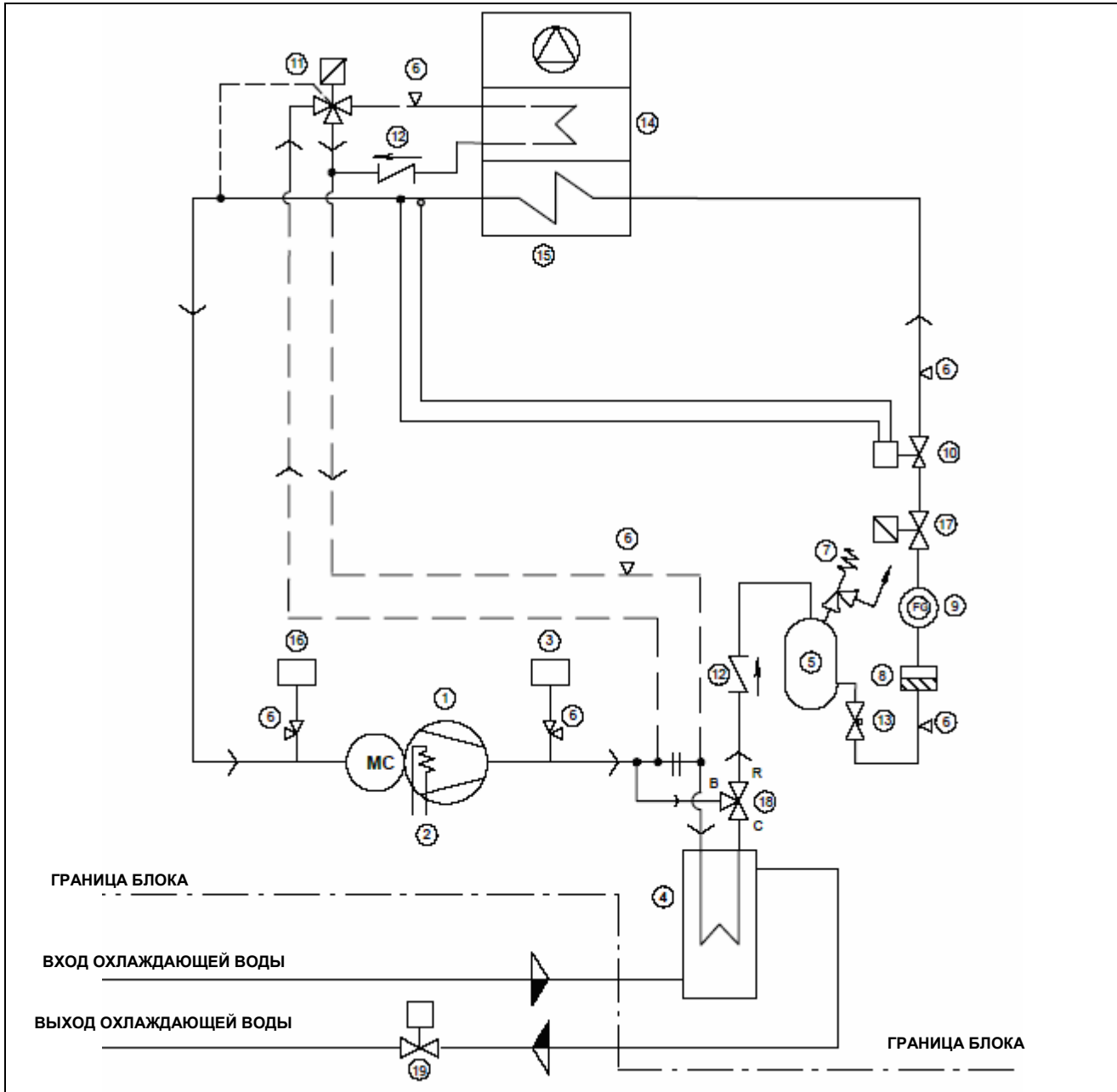
Рис. 4. Liebert Hiross HPM Sxx U/O W
