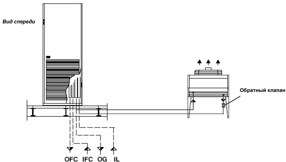
Рис. 9. Соединения контура охлажденной воды и хладагентного контура блоков Liebert Hiross HPM SxxxD, MxxxD и LxxxD
