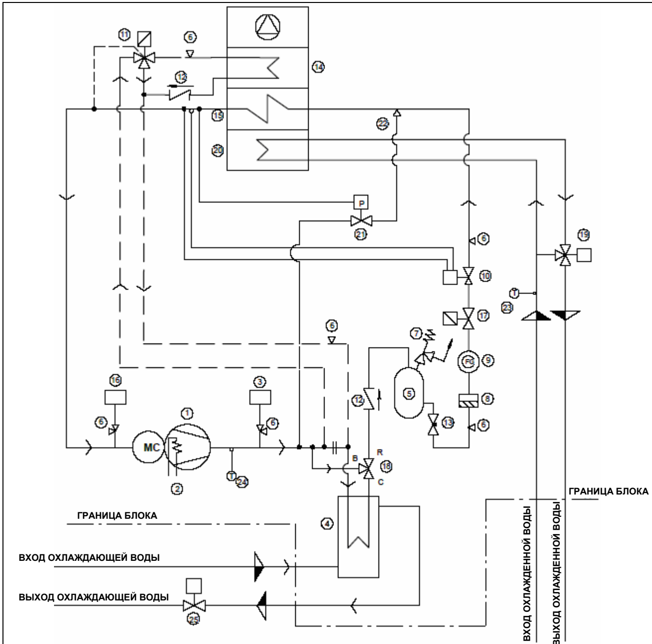
Рис. 15. Liebert Hiross HPM Sxx U/O H
