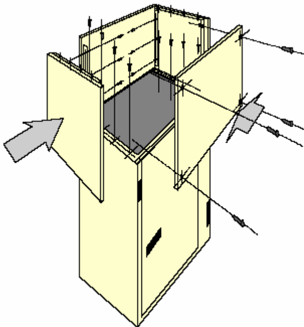
Рис. 7. Удлинительный воздуховод
