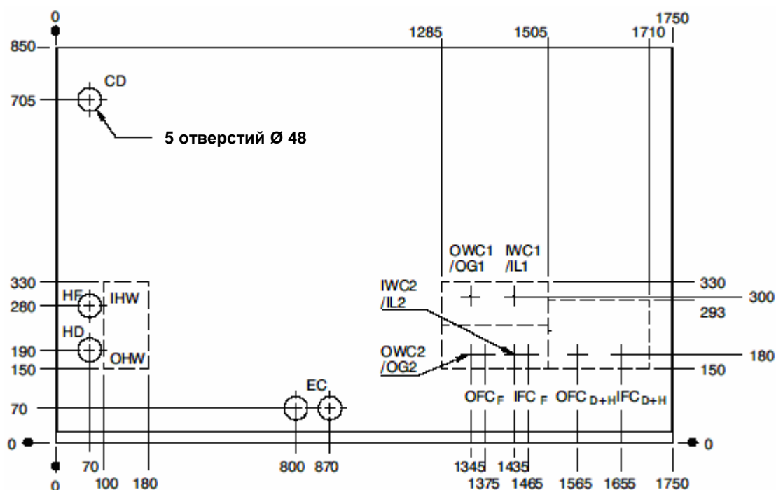
Рис. 5. Хладагентные, водяные и электрические соединения Liebert Hiross HPM M31...66
