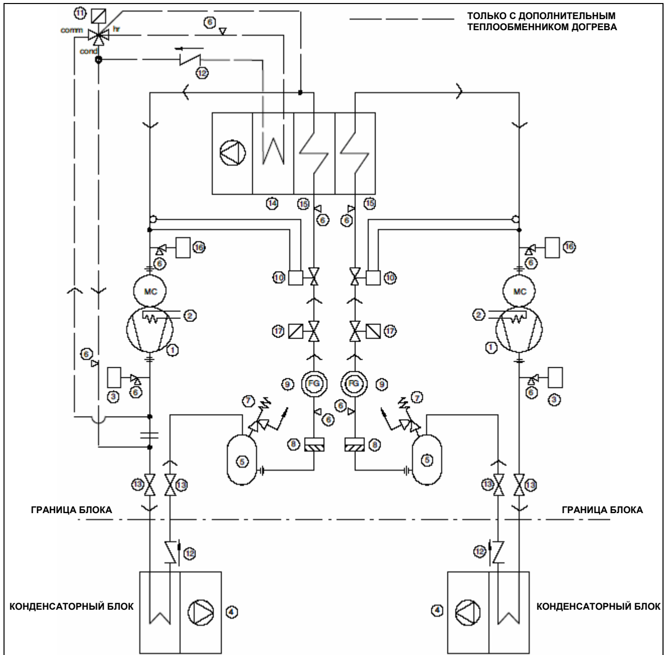
Рис. 3. Liebert Hiross HPM L83 – 99 U A
