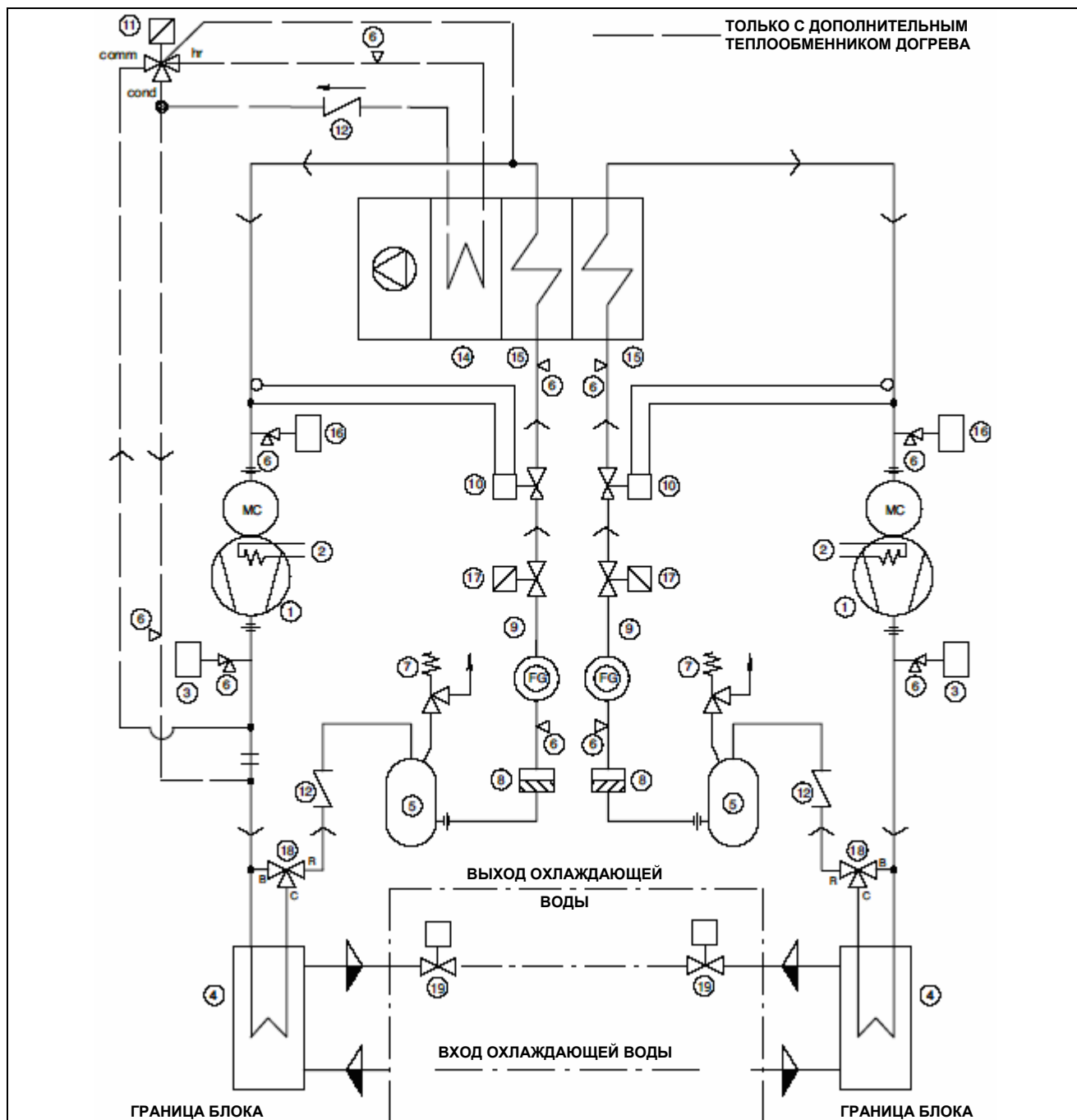
Рис. 7. Liebert Hiross HPM L83 - 99 U W
