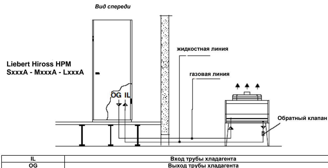
Рис. 7. Соединения хладагентного контура
