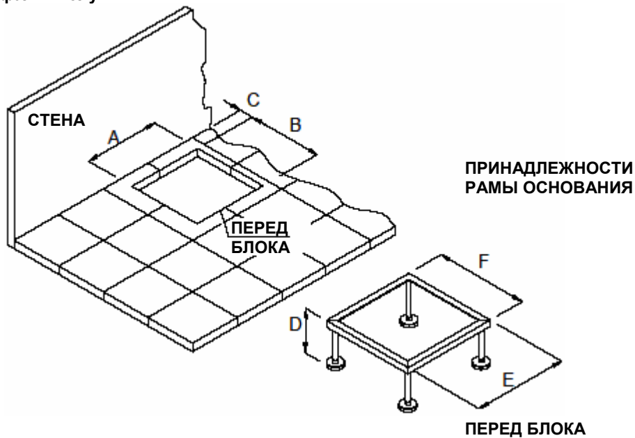
Рис. 6. Отверстие в фальшполу
