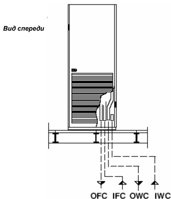
Рис. 9. Соединения контура охлажденной воды и хладагентного контура блоков Liebert Hiross HPM SxxxD, MxxxD и LxxxD
