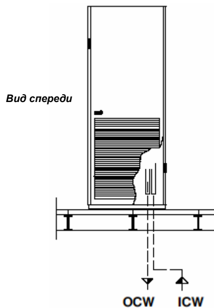
Рис. 8. Соединения контура охлажденной воды Liebert Hiross HPM SxxxF/H, MxxxF/H и LxxxF/H
