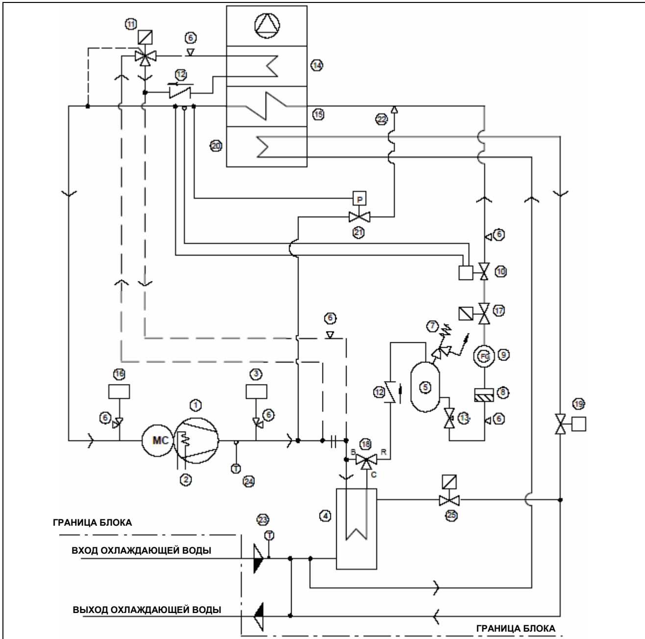
Рис. 9. Liebert Hiross HPM M25 - 47 U/O F
