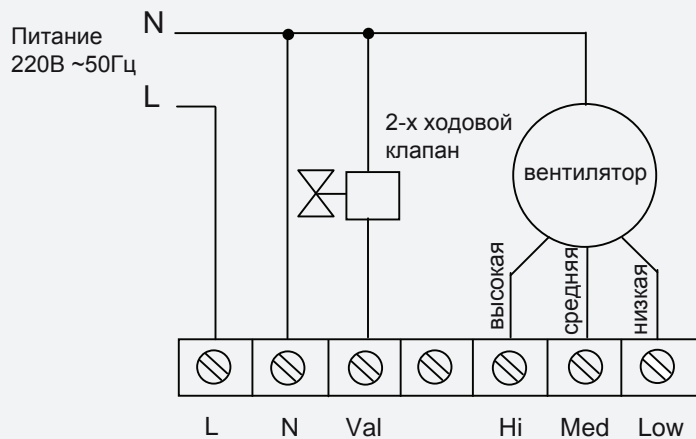
проводной термостат LZ-FBPW2
