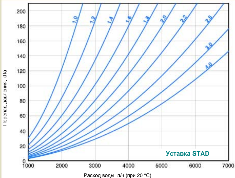
График 2: Перепад давления на гидравлической системе HG5C при различных значениях уставки STAD теплообменника
