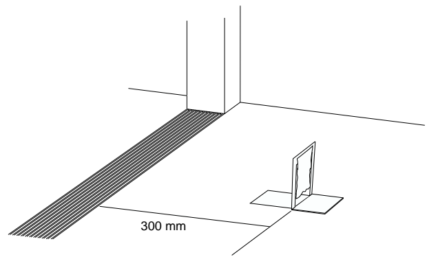
Afstelgereedschap plaatsen
