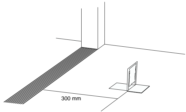
Asetustyökalan sijoitus
