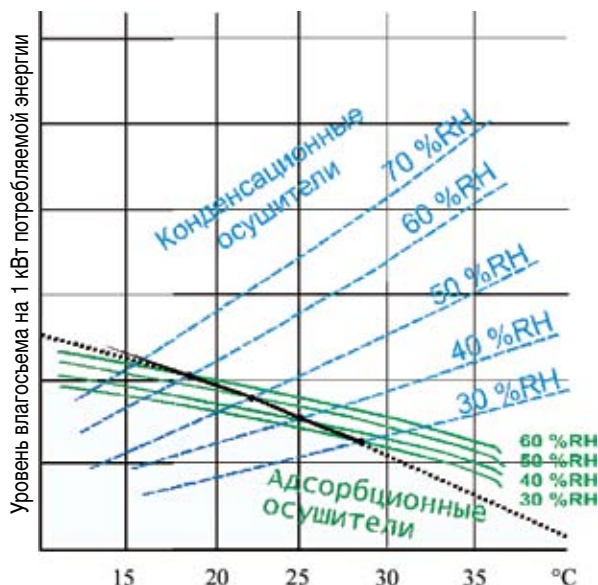
Рис. 4. Эффективность работы осушителей разного типа
