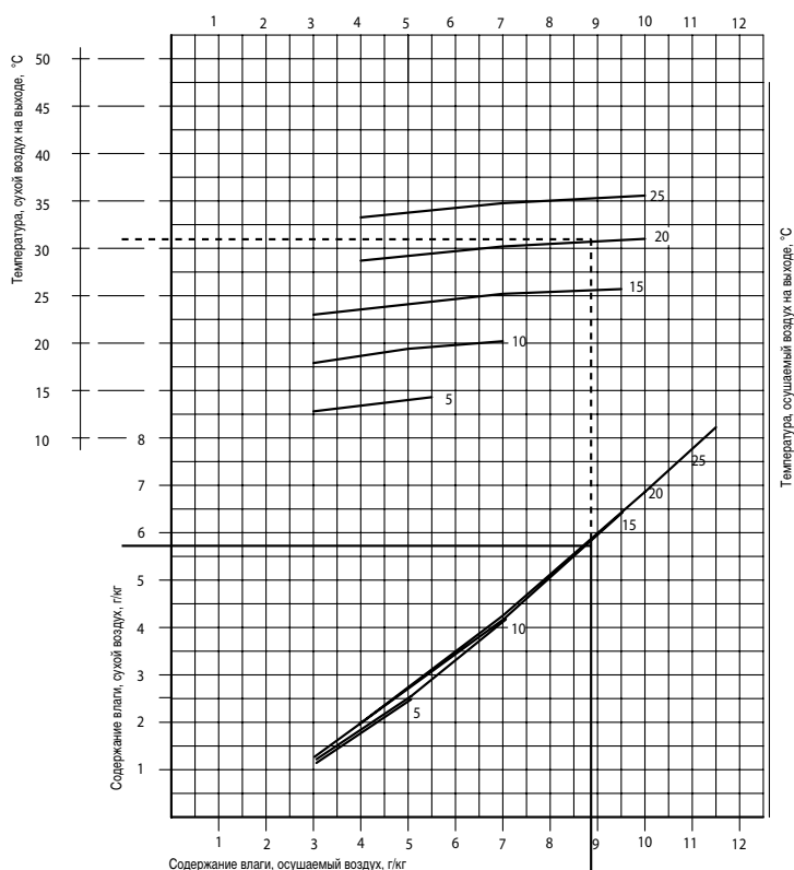
Рис. 21. Пример расчета производительности для осушителя AD 120 В.
