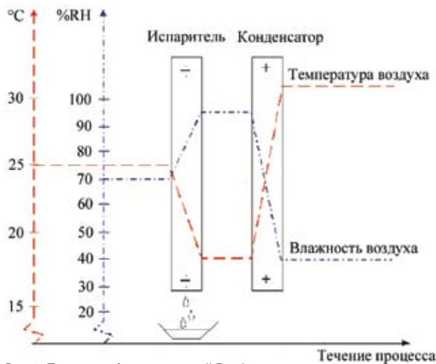
Рис. 6. Принцип работы осушителей Dantherm
