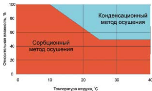
Рис. 5. Преимущественные области использования различных методов осушения
