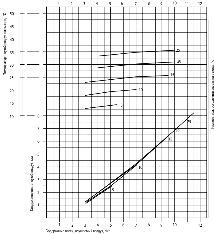
Рис. 19. Кривые влагосъема для осушителя серии AD 290 В.
