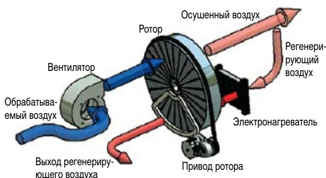
Рис. 7. Принцип действия осушителей AD 120...400 В.
