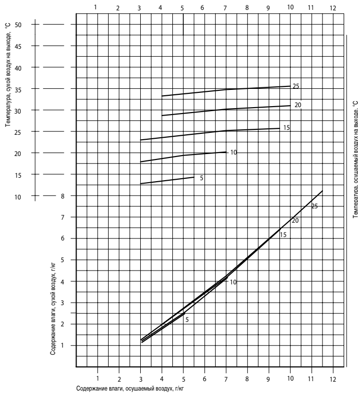
Рис. 20. Кривые влагосъема для осушителя серии AD 400 В.
