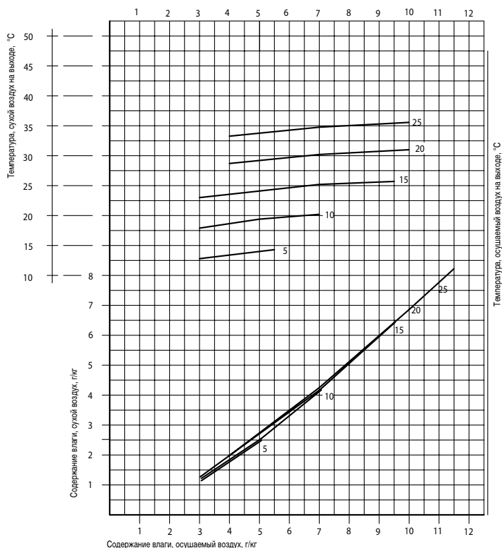
Рис. 18. Кривые влагосъема для осушителя серии AD 240 В.
