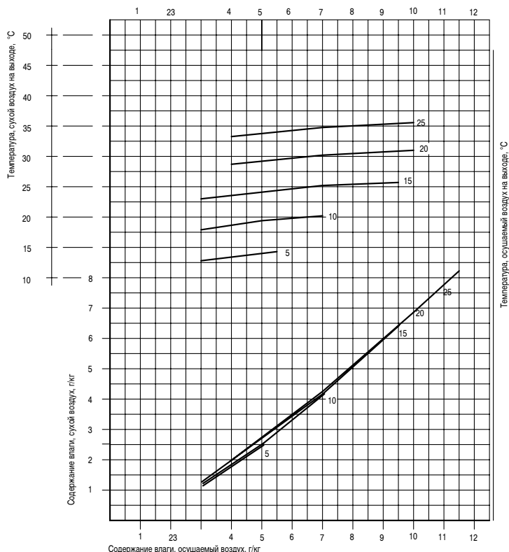
Рис. 17. Кривые влагосъема для осушителя серии AD 120 В.
