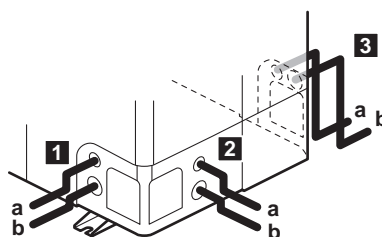
a Проводка управления
