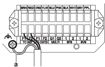
a Заземление
