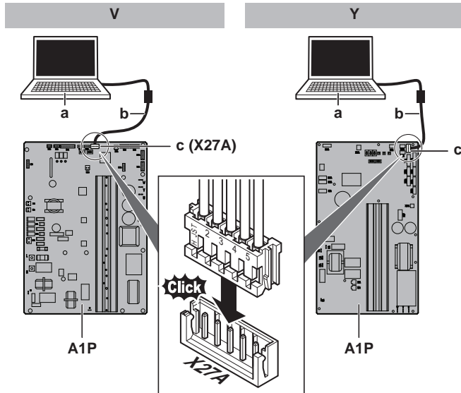
▲ 17-1 1 фаза (V)
