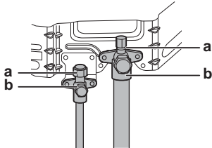
a Сервисное отверстие b Запорный клапан
