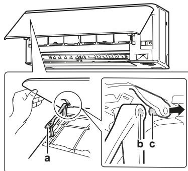
a Важіль b Паз c Держак
