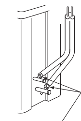
Проверьте места для монтажа блока внешней установки
