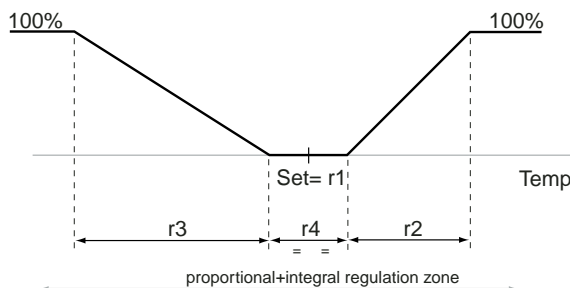
Valvola riscaldamento-raffredd. / Heating-Cooling Valve -Fig. 24-
