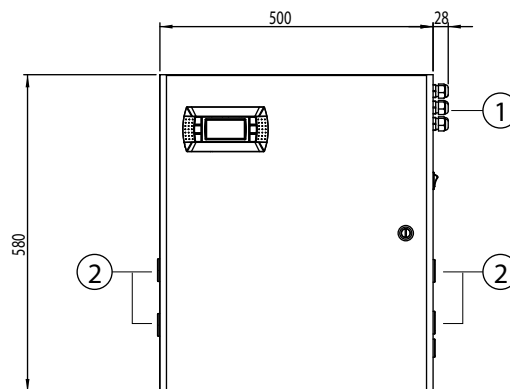
Изображение шкафа, отверстие впуска воздуха и воды, вод сбоку
