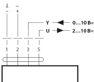
Схема электрических соединений
