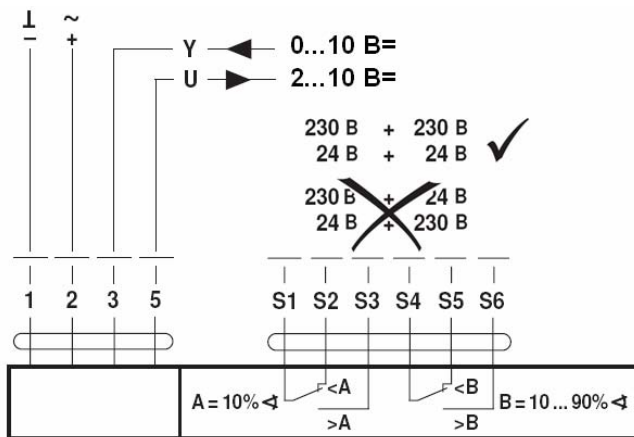
Схема подключения
