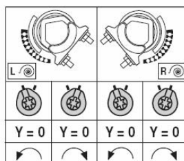
Направление вращения
