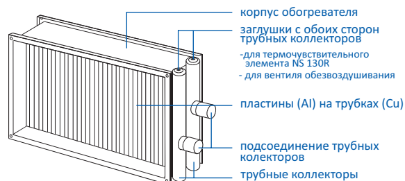
Рис. 2 Конструкция обогревателя.
