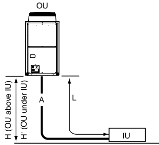
Fig.IV-1-(1)A : PUHY Piping Design
