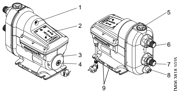
Рис. 1. Внешний вид Grundfos SCALA2
