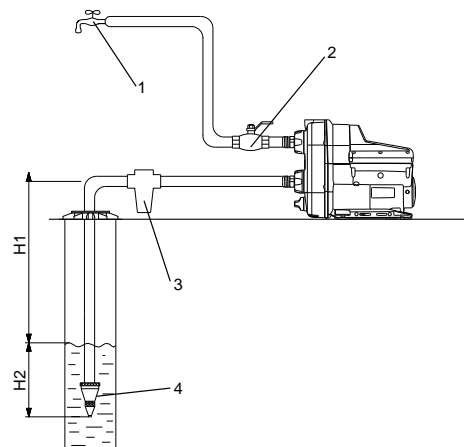
Рис. 3. Подача воды из колодца / скважины
