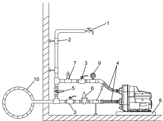
Рис. 2. Повышение давления воды из магистрального трубопровода
