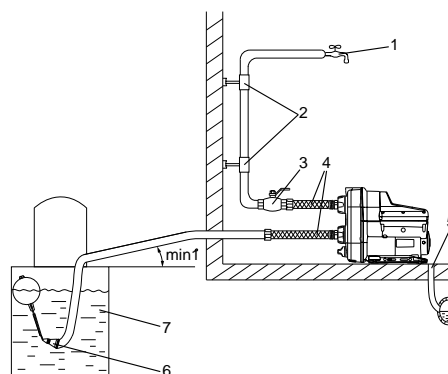
Рис. 4. Подача воды из резервуара
